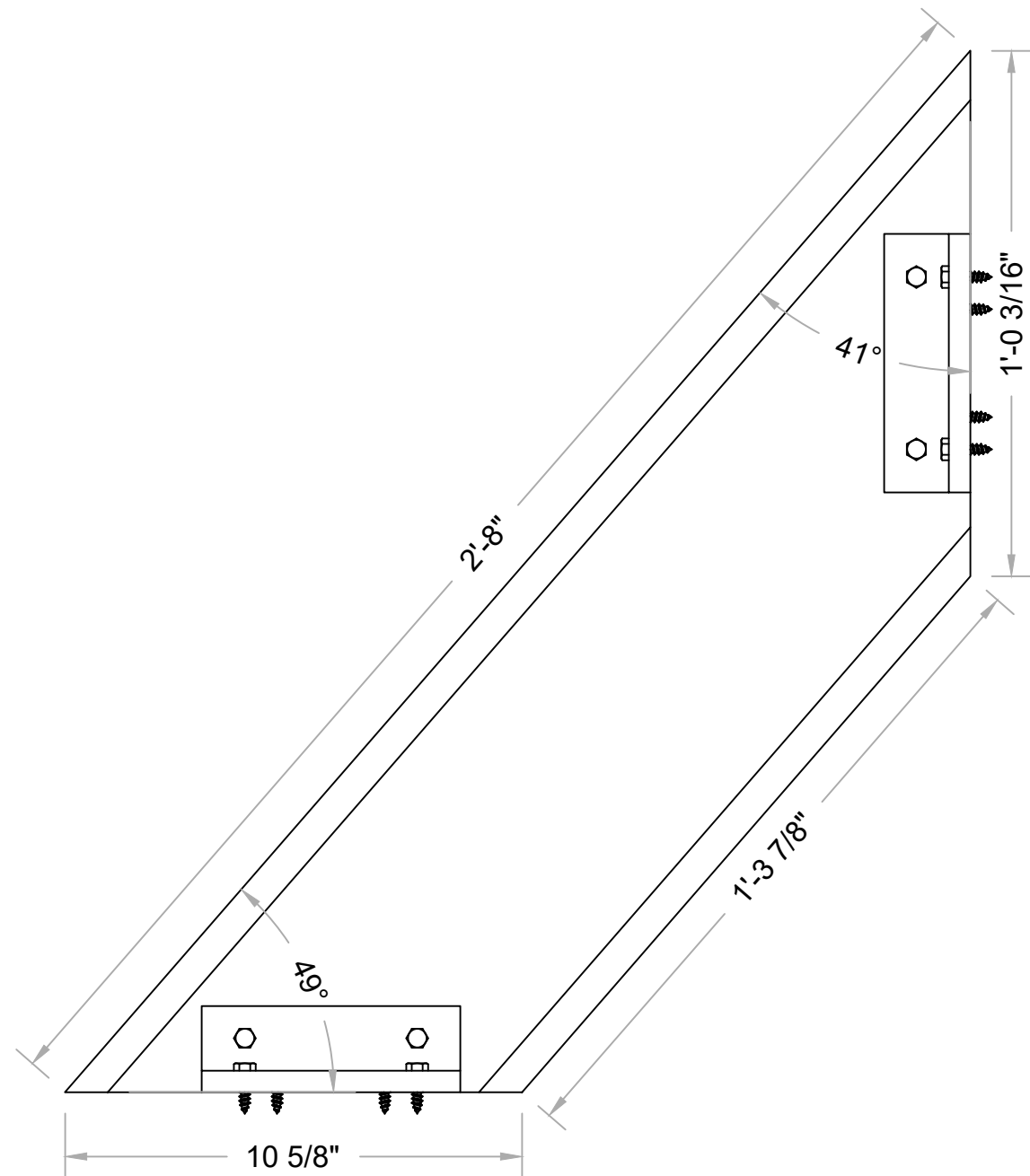
3 RIGHT Scale: 3" = 1'-0"
