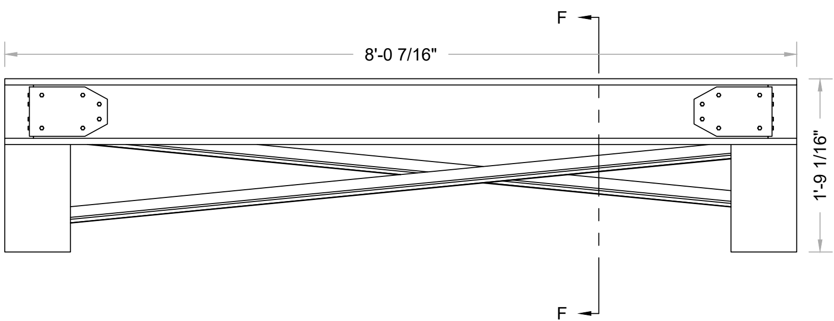
2 FRONT Scale: 1" = 1'-0"
