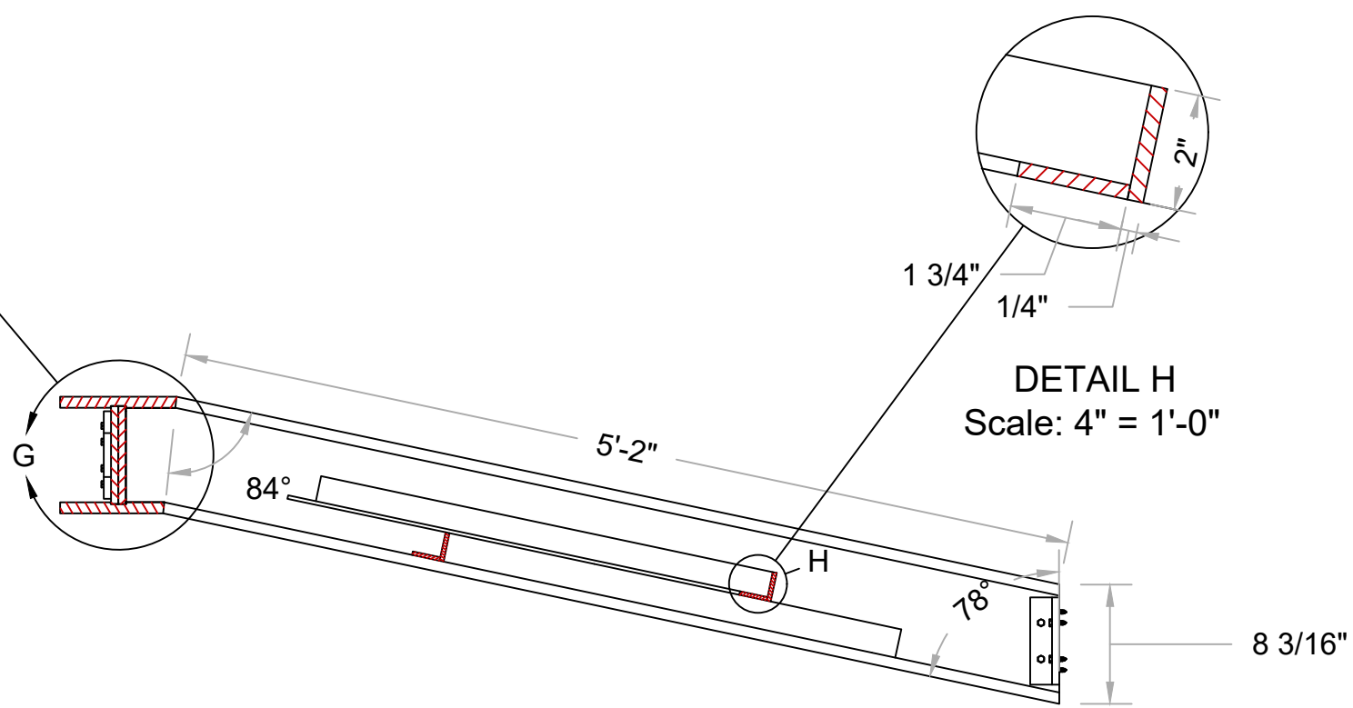
3 SECTION F-F Scale: 1" = 1'-0"
