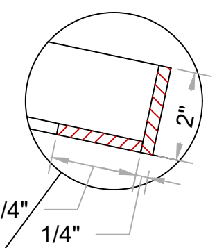
DETAIL H Scale: 4" = 1'-0"
