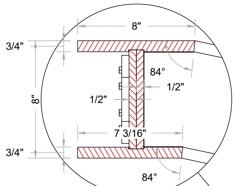
DETAIL G Scale: 3" = 1'-0"
