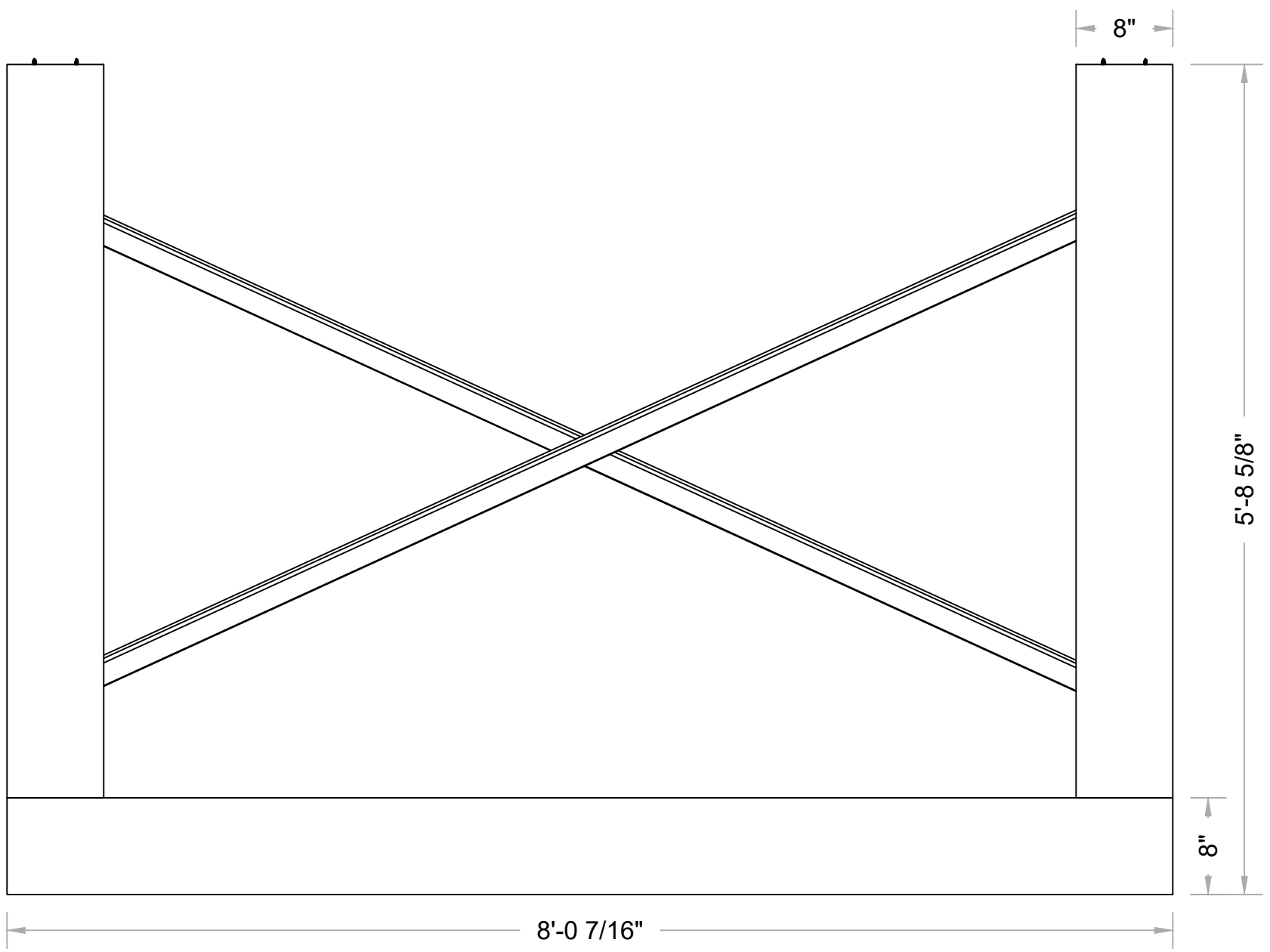
1 TOP Scale: 1" = 1'-0"
