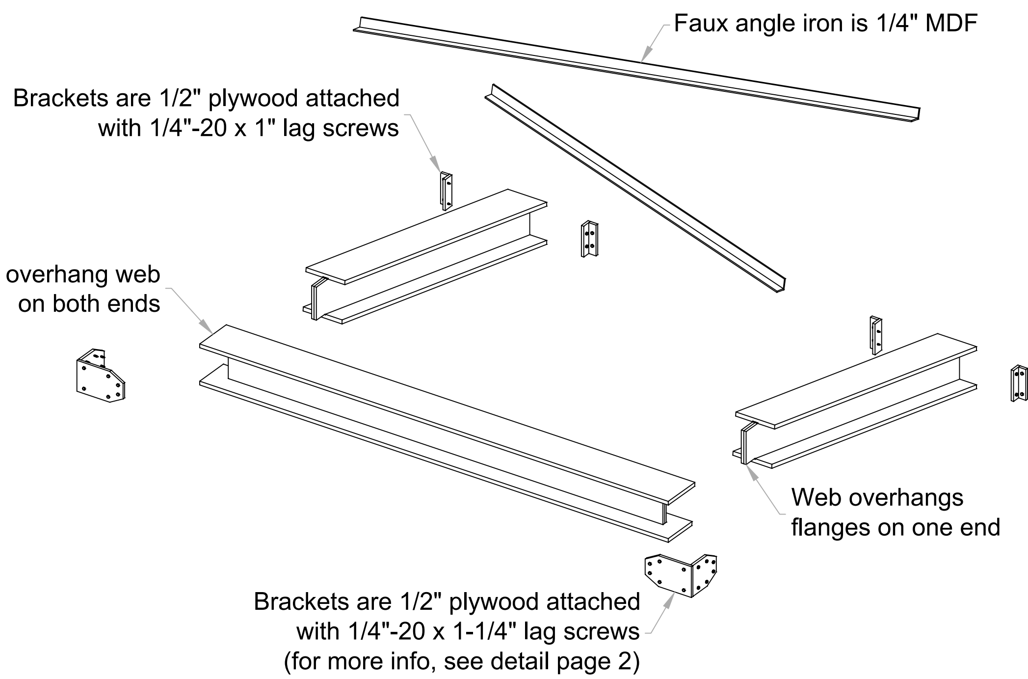
5 SEPARATED ISO Scale: NTS
