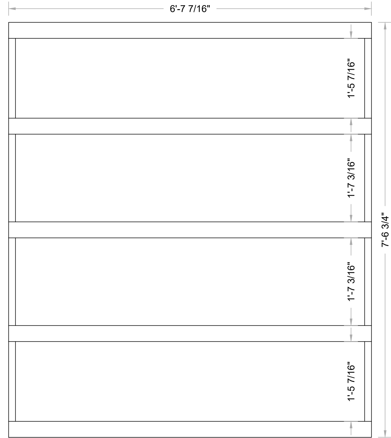
1 TOP Scale: 1" = 1'-0"
