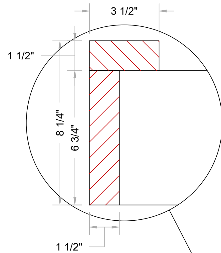
DETAIL I Scale: 4" = 1'-0"
