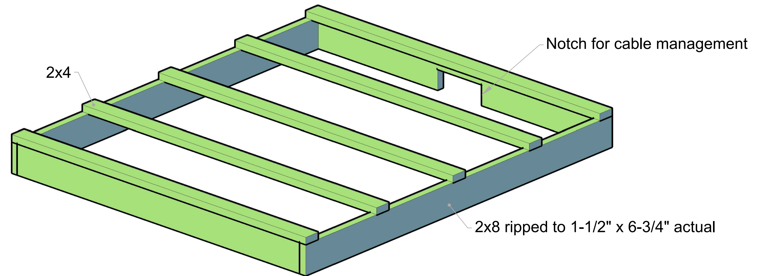
5 FRONT ISO Scale: NTS
