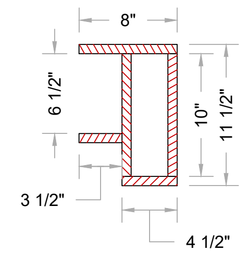
2 SECTION K-K Scale: 1-1/2" = 1'-0"
