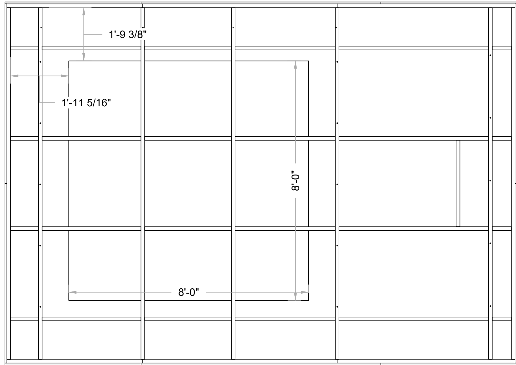
1 TOP Scale: 1/2" = 1'-0"
