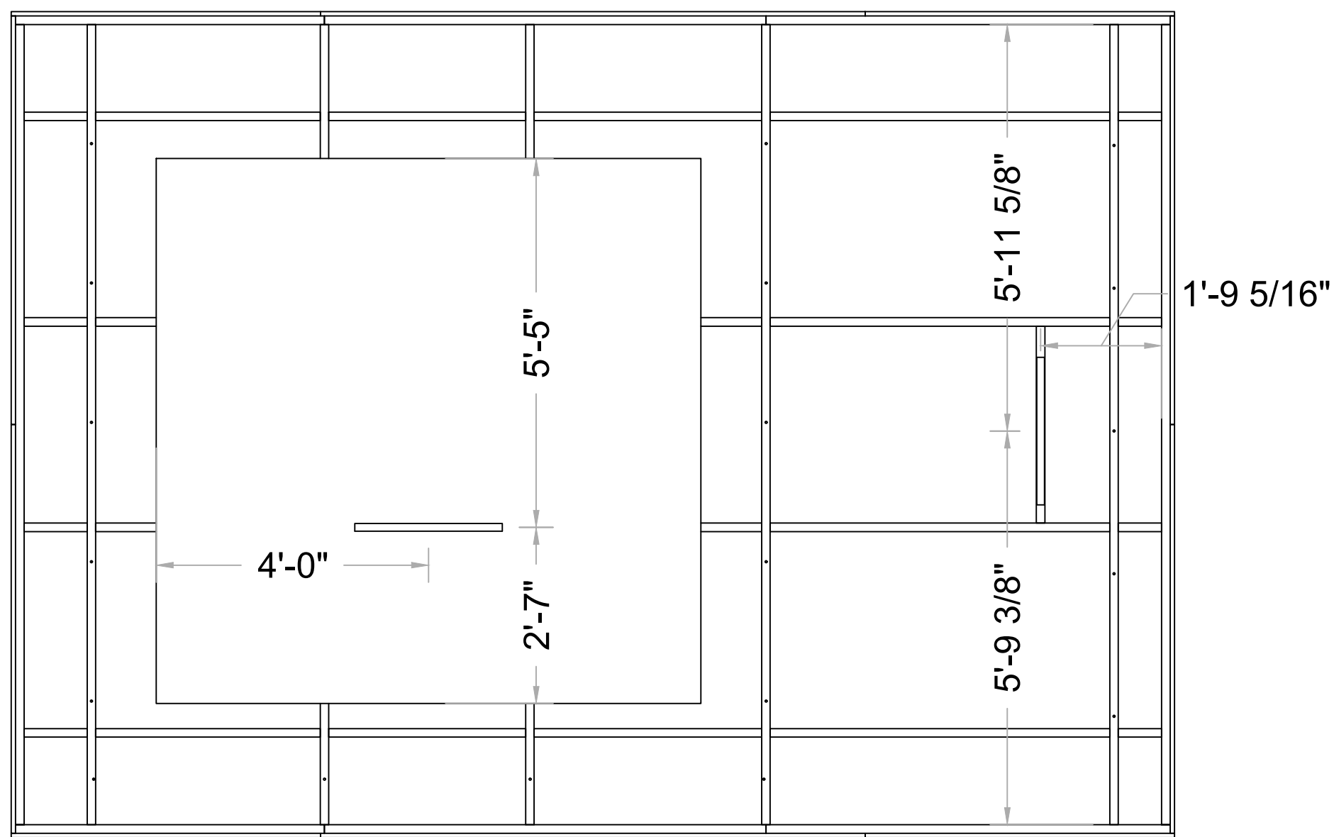
3 BOTTOM Scale: 1/2" = 1'-0"
