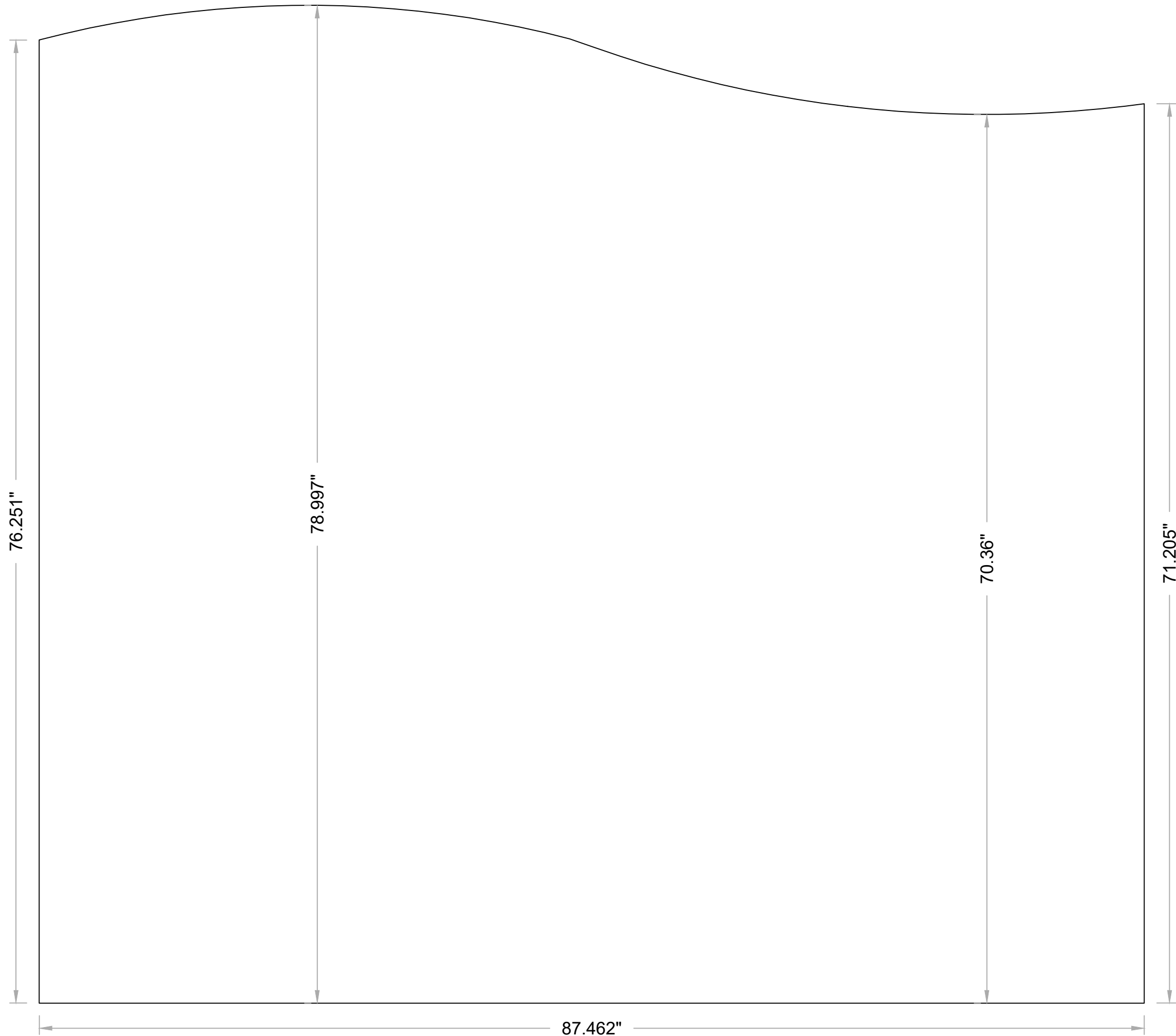
1 FRONT SKIN Scale: 1-1/2" = 1'-0"
