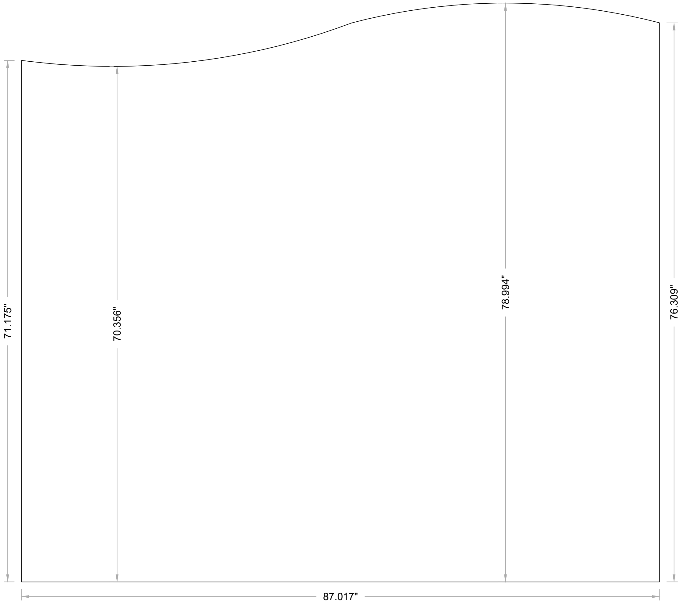
1 BACK SKIN Scale: 1-1/2" = 1'-0"
