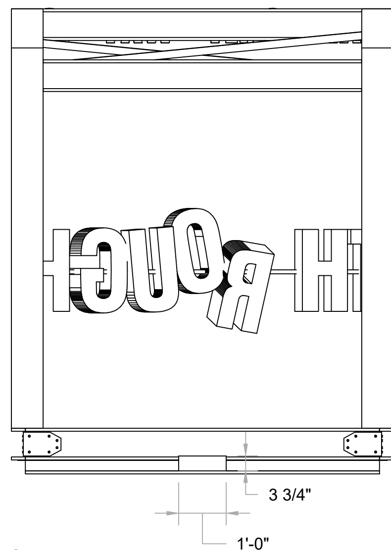
4 BACK Scale: 1/2" = 1'-0"
