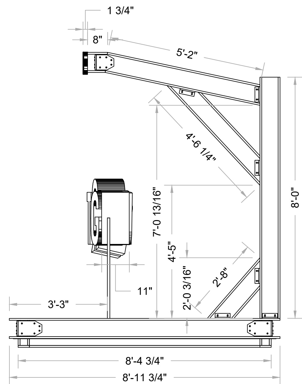
3 RIGHT Scale: 1/2" = 1'-0"
