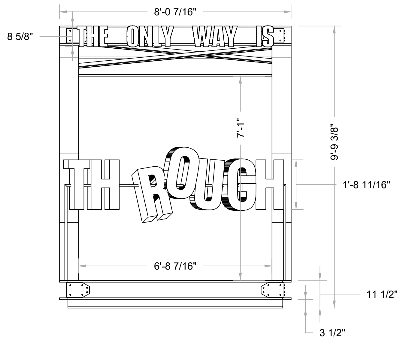
2 FRONT Scale: 1/2" = 1'-0"
