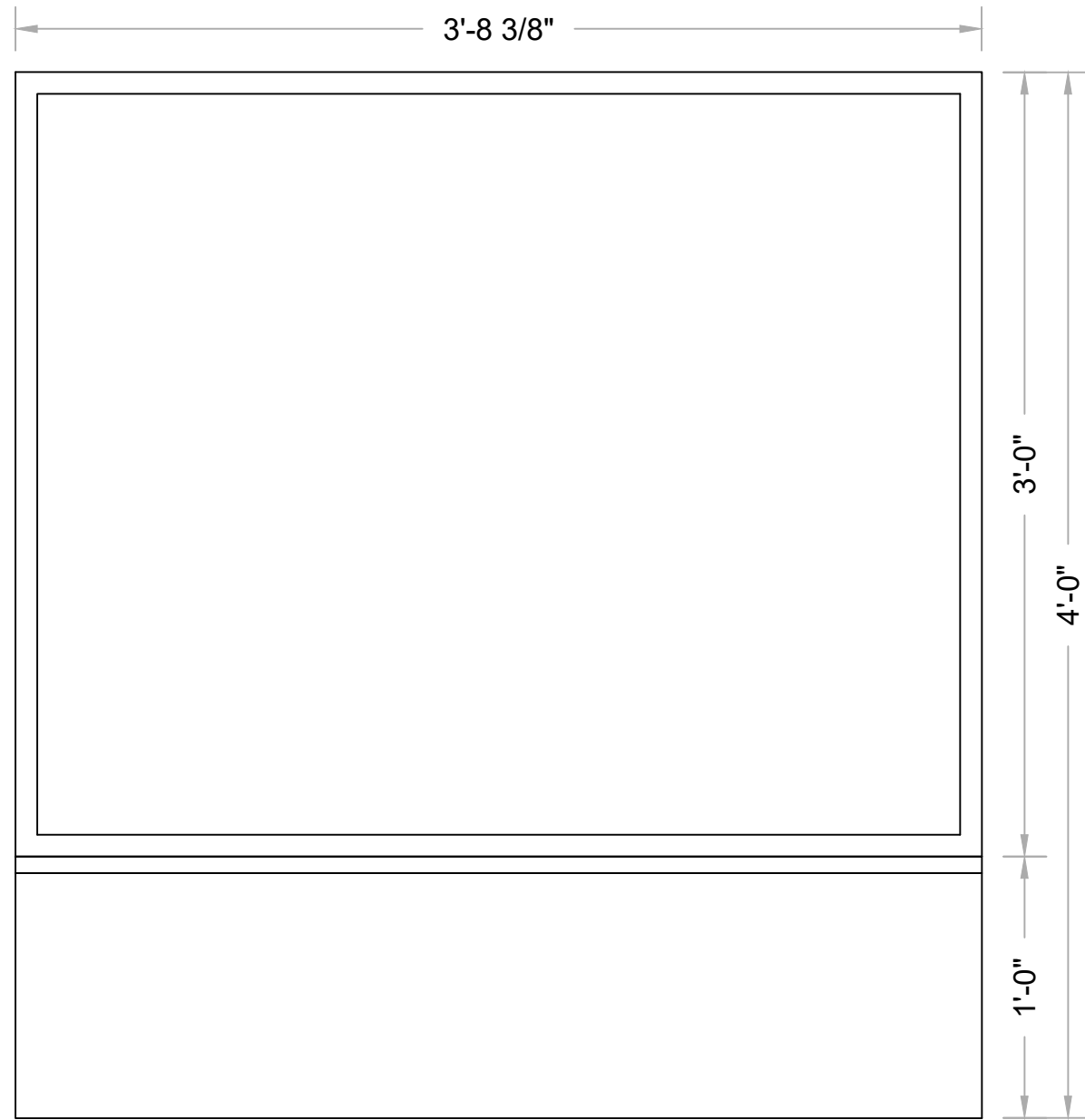
2 FRONT Scale: 1/2" = 1'-0"
