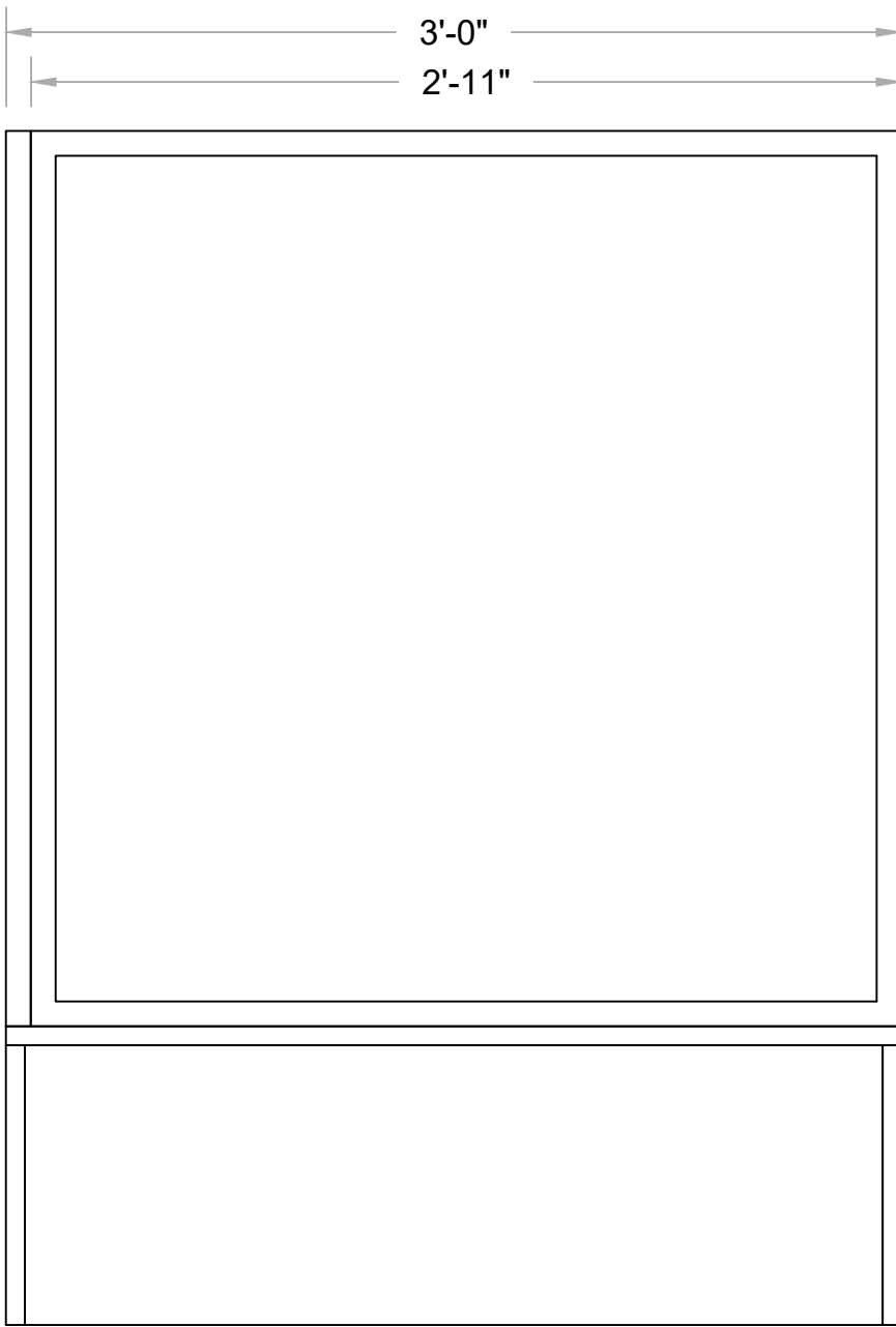
3 RIGHT Scale: 3/8" = 1'-0"
