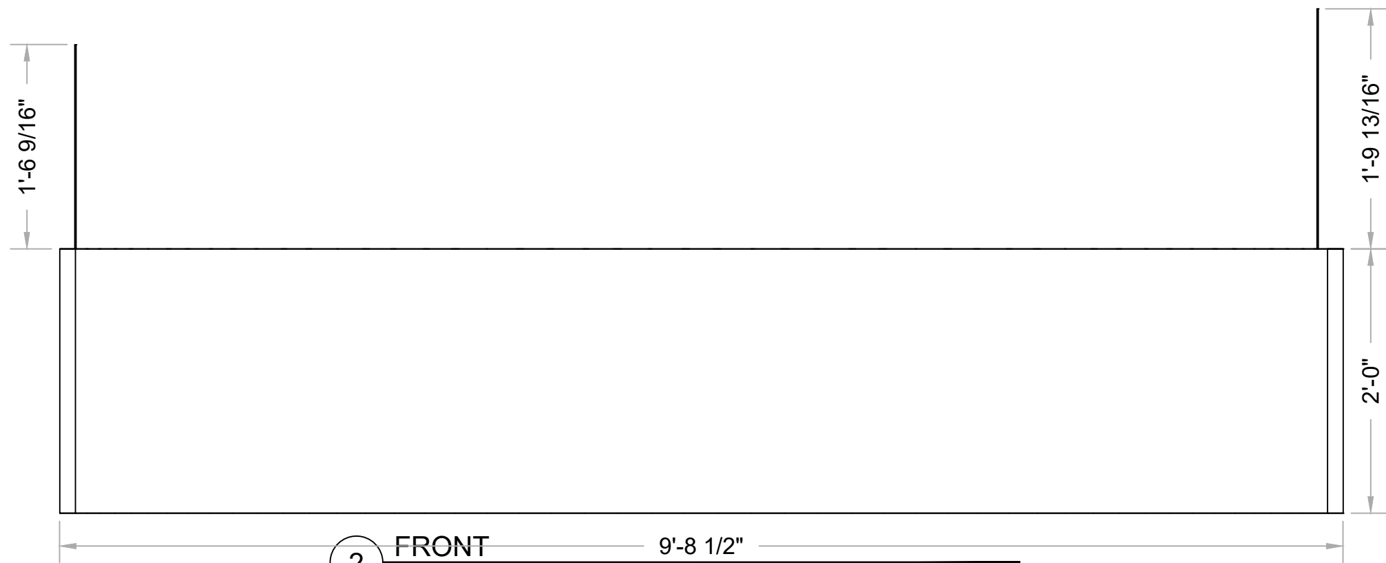
2 FRONT Scale: 1" = 1'-0"
