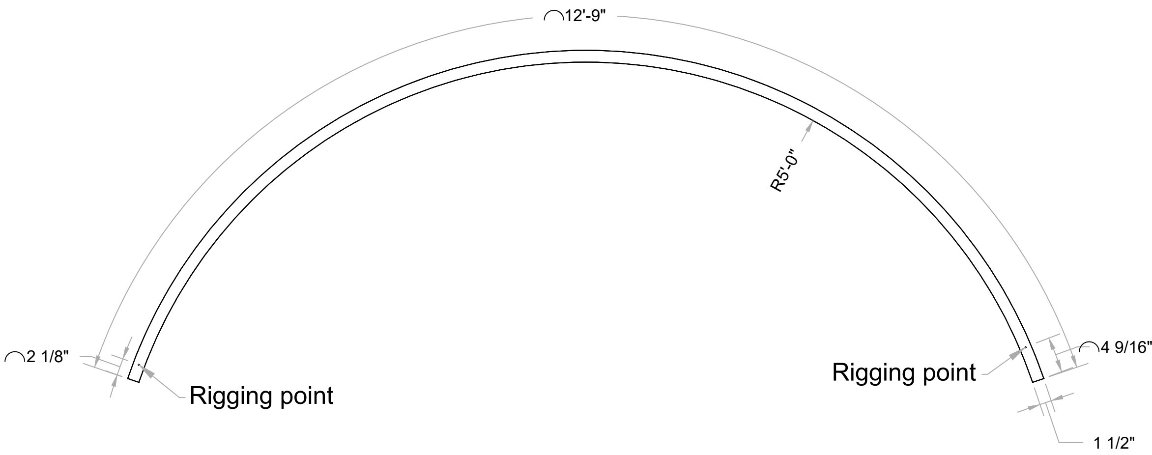
1 TOP Scale: 1" = 1'-0"
