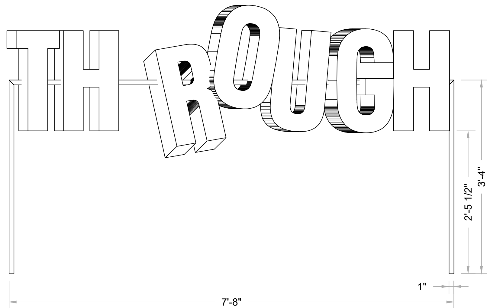
2 FRONT Scale: 1" = 1'-0"
