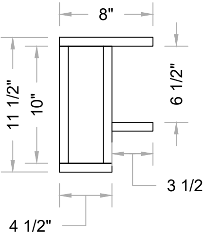
3 RIGHT Scale: 1-1/2" = 1'-0"
