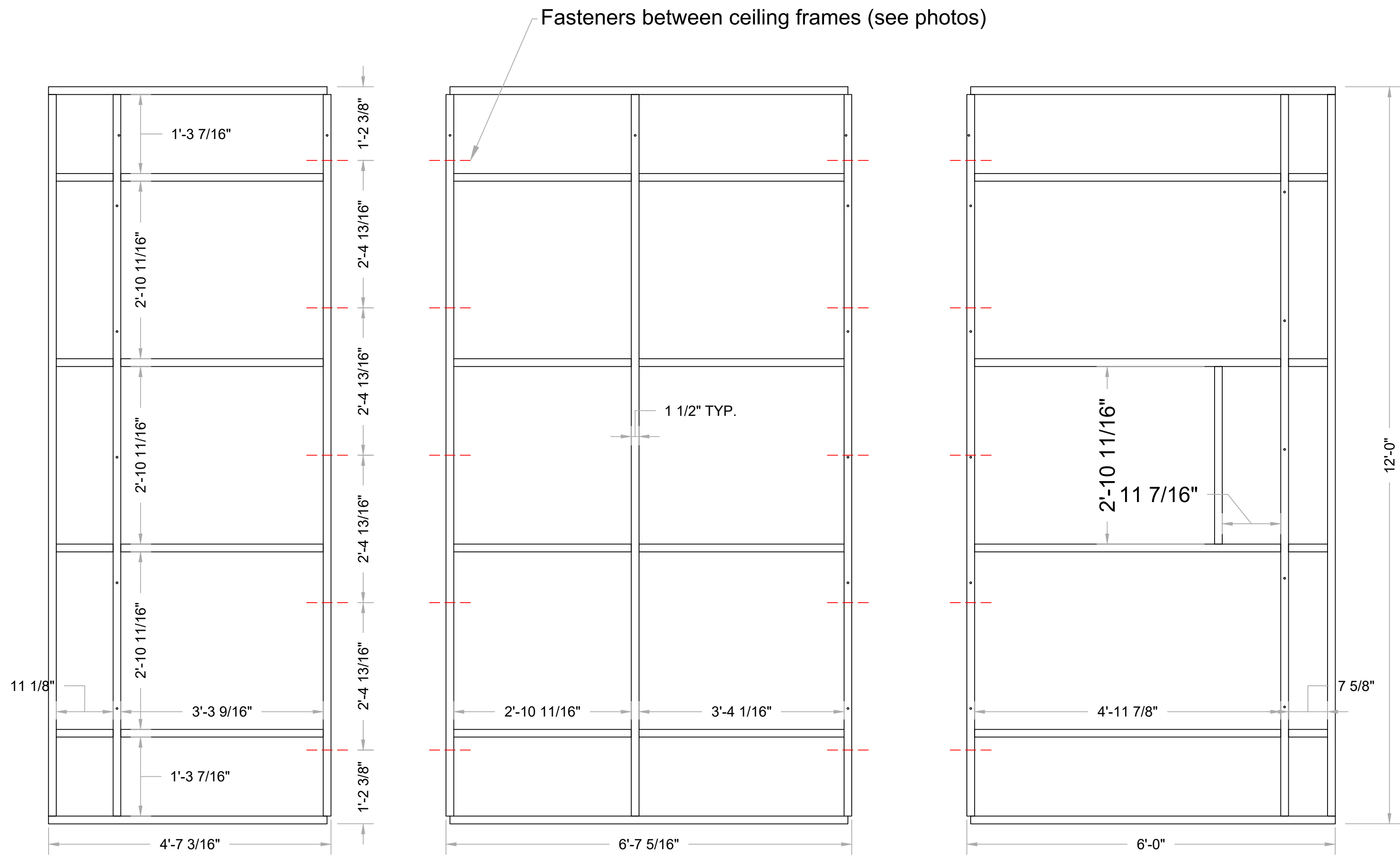
1 TOP Scale: 3/4" = 1'-0"
